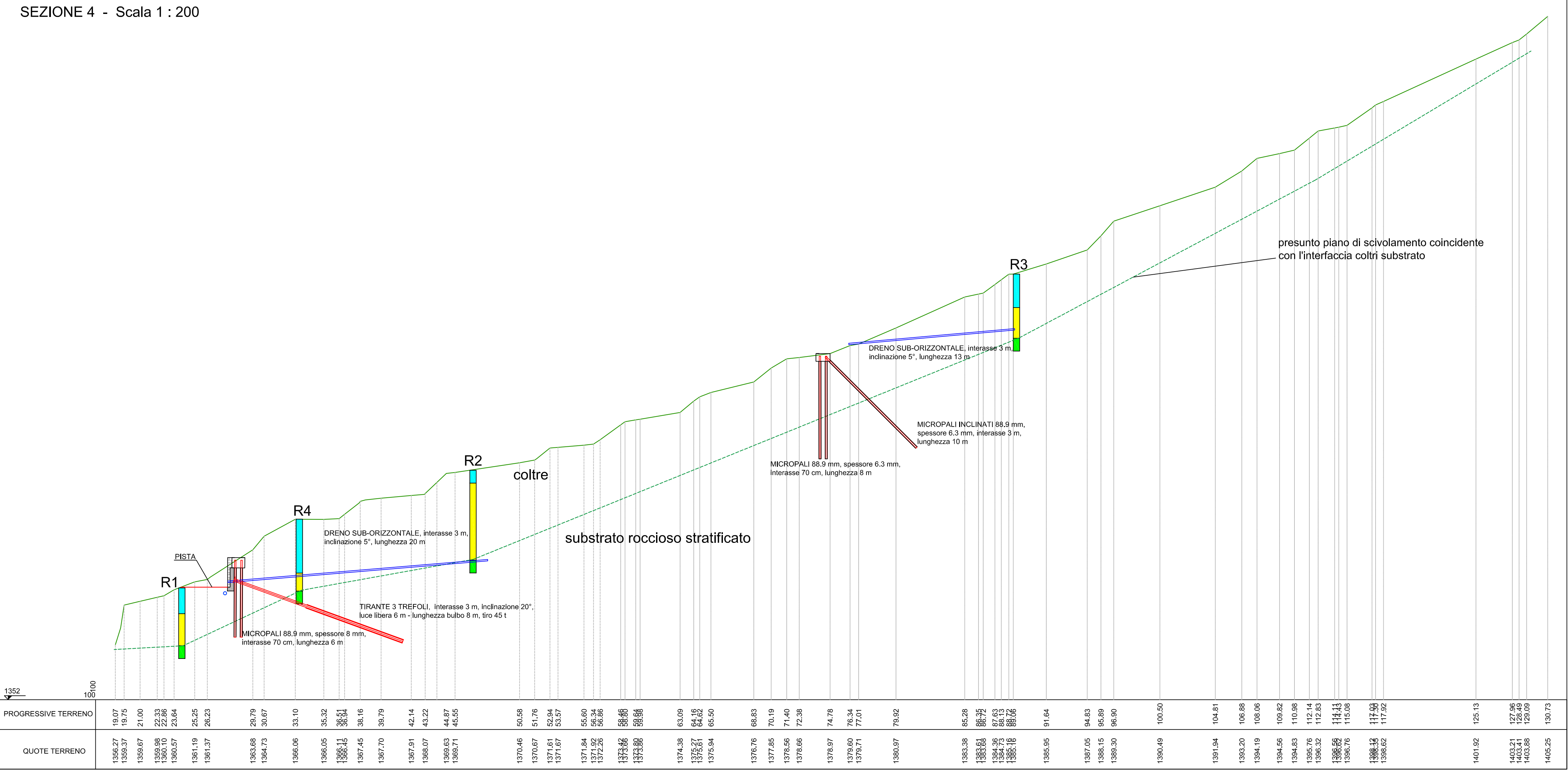
SEZIONE 5 - Scala 1 : 200
